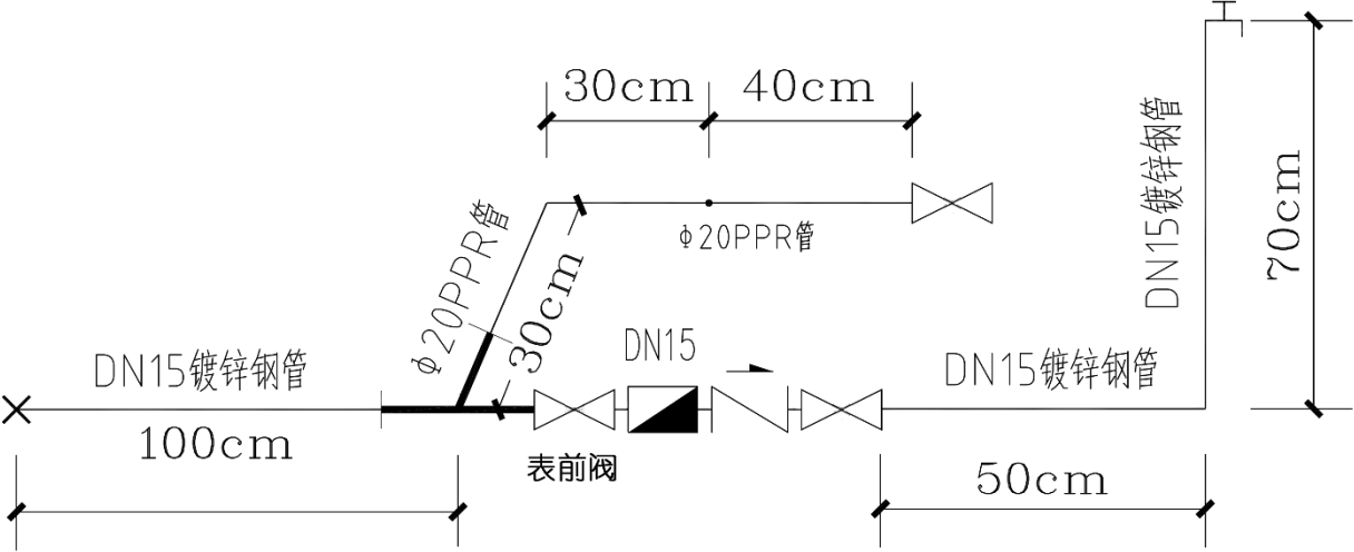
安装示意图:
