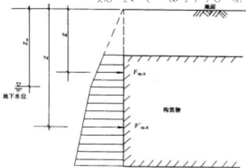
图 4.2.4 侧壁上的主动土压力分布图
